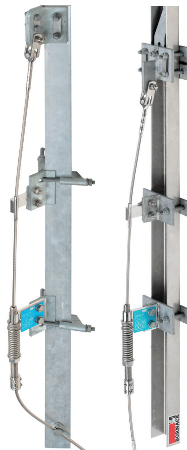
Steigschutzsystem SSE Variante Eckstiel: gesamtes Spannseil SSE Gabelterminal oben, Seil, Seilführung, Spannvorrichtung, Eckstiel.
